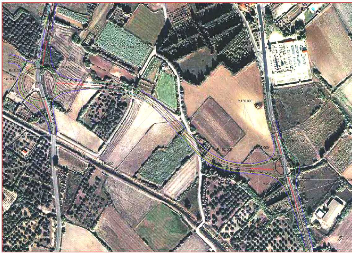
ORTOFOTO CON TRACCIATO STRADA DI PROGETTO
